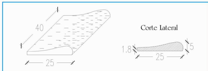
BORDE OCEANICO 40 cm. x 25 cm.
